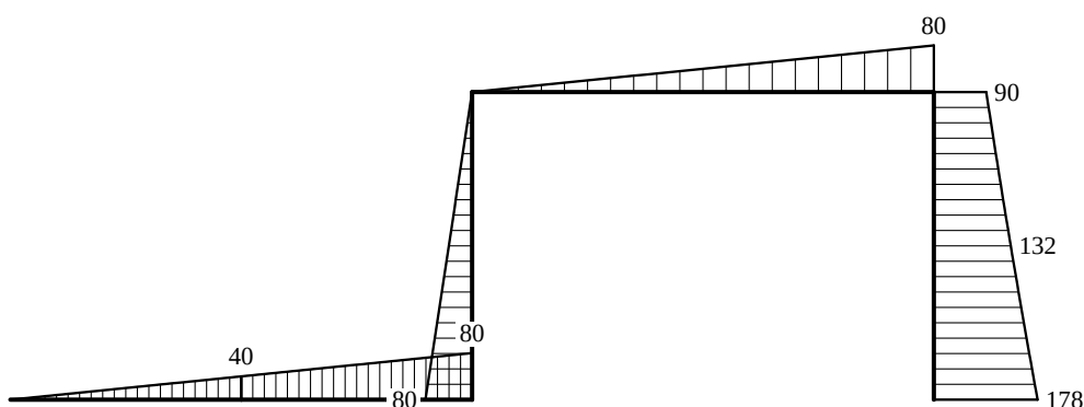
Схема 4 — эпюра M, кН·м
